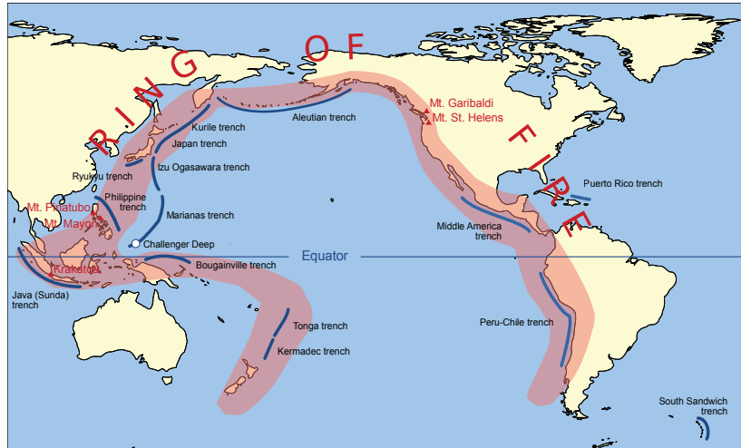
Gambar 1.18. Indonesia sebagai Salah Satu Negara Kawasan Ring of Fire
