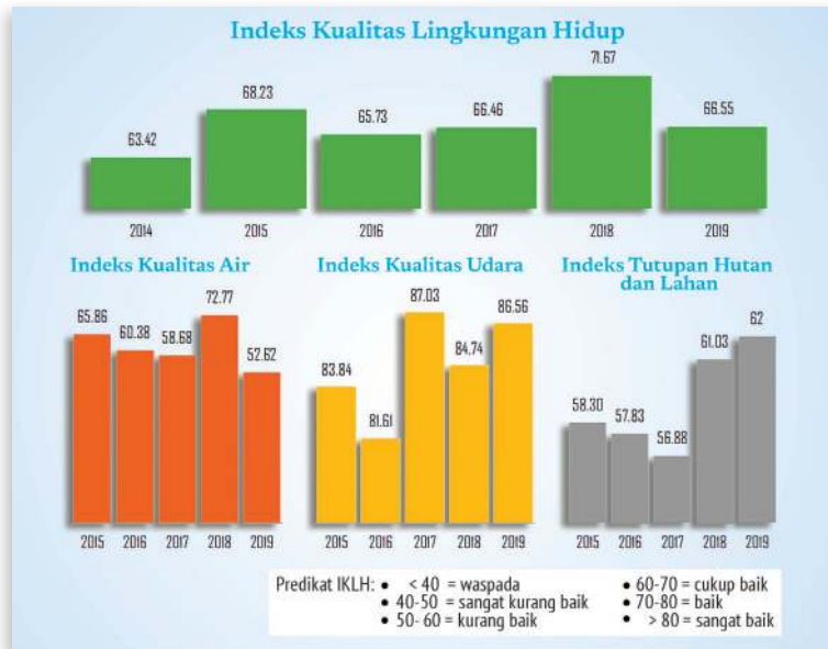
Gambar 3.8. Capaian IKLH, IKA, IKU dan IKTL Tahun 2015 – 2019
