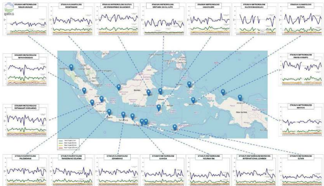
Gambar 1.8.. Peta Tren Curah Hujan Indonesia
