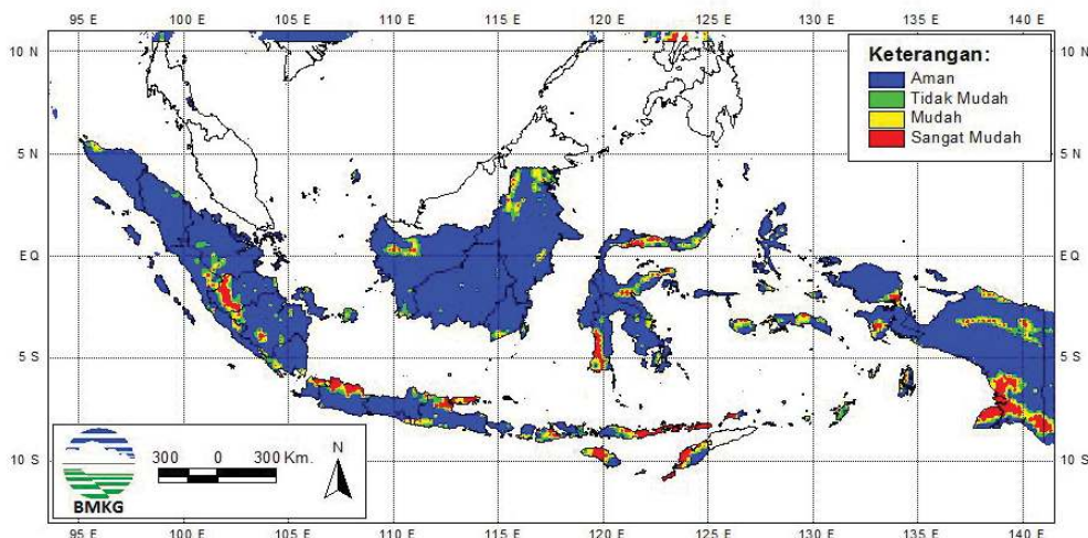
Gambar 4.21. Peta Potensi Kemudahan Terjadinya Kebakaran Ditinjau dari Analisa Parameter Cuaca Sumber: bmkgo.id (2020)
