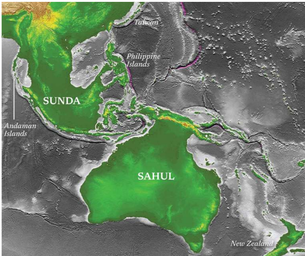
Gambar 1.11. Letak Geologis Indonesia di antara Dua Dangkalan/Paparan Sumber: PECKHAMIA May 2010
