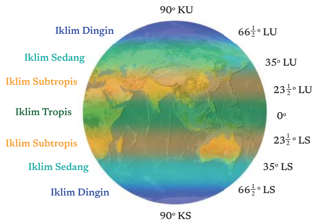
Gambar 1.3. Pembagian Iklim Matahari
